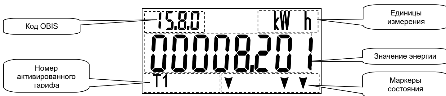
Рис. 7: Пример индикации регистра энергии (тестовый режим)
