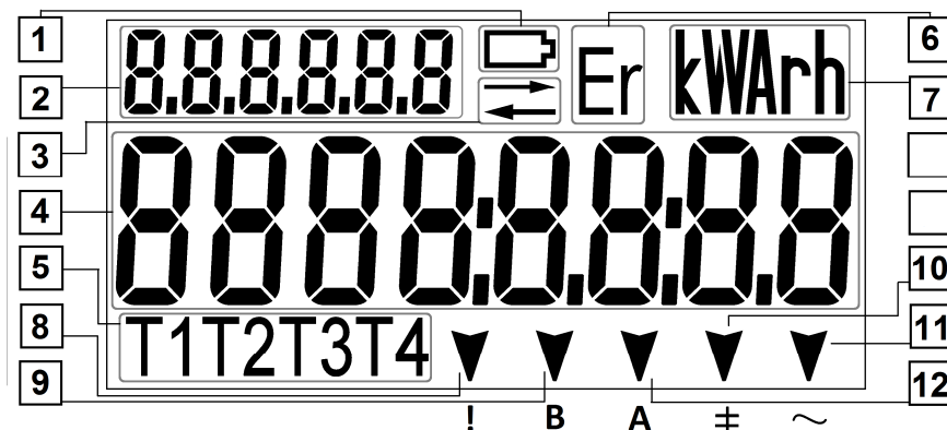
Рис. 3: Сегменты и поля ЖКИ счетчика G1M
