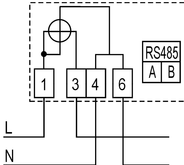
Рис. 8: Схема подключения счетчика G1M - один элемент измерения тока (шунт) и интерфейс связи RS485
