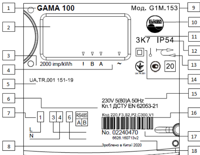
Рис. 2: Щиток счетчика G1M
