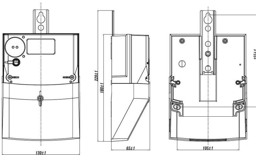
Рис. 9: Размеры счетчика и отверстия крепления
