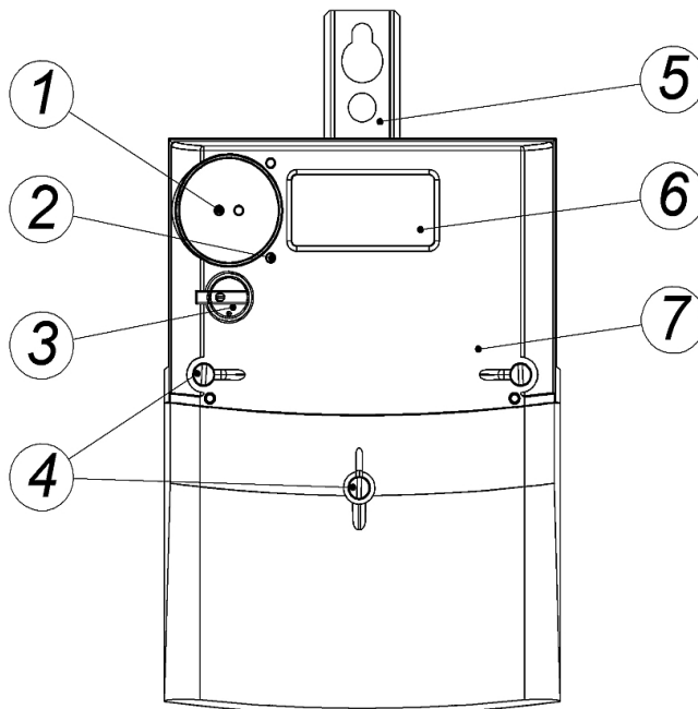
Рис. 1: Внешний вид счетчика G1M
